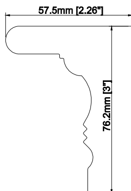
3" Deco Sill Frame
